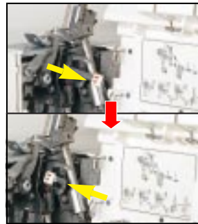
SISTEMA AUTOMATICO DI INFILATURA DEL CROCHET INFERIORE
